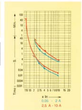
5 x 20 Temporizado
