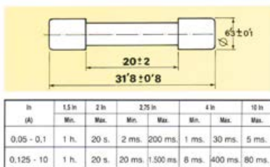
5 x 20 Rápido
