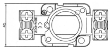
Base D03 100A 400V~
