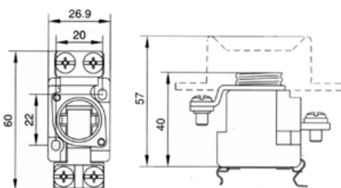
Base D02 63A 400V~
